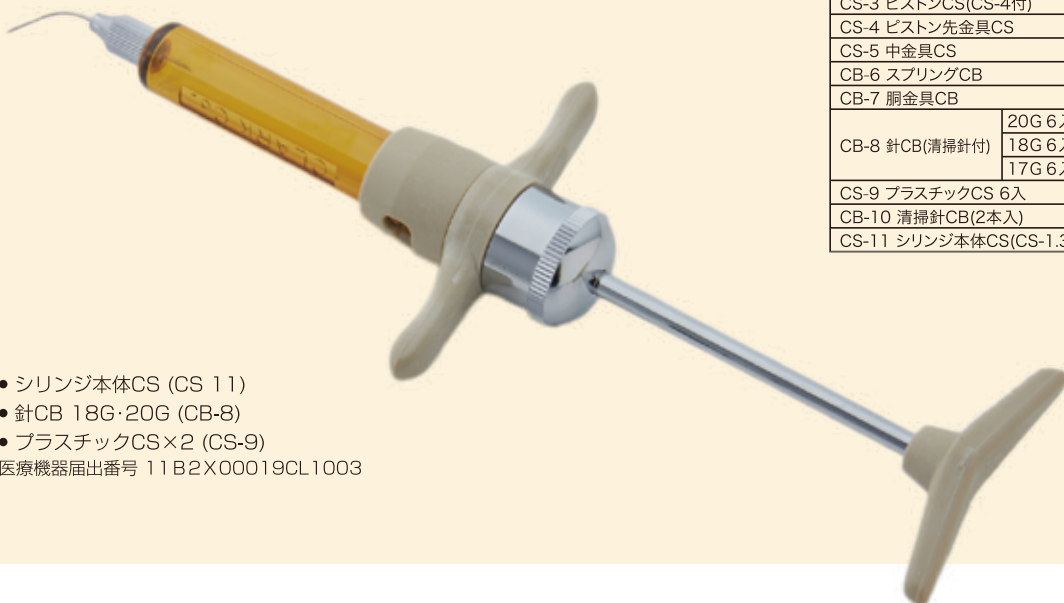
Pカートリッジシリンジ部品
